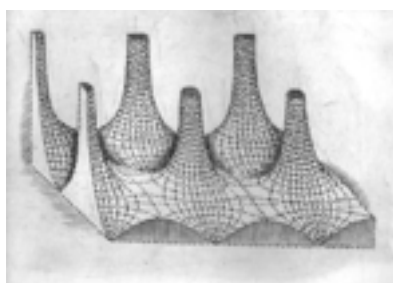
Fig. 28. Sinus-amplitude function
