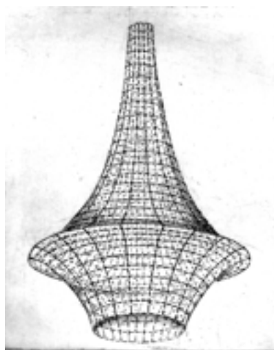
Fig. 21. Pseudo-sphere
