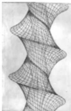
Fig. 22. Dini surface
