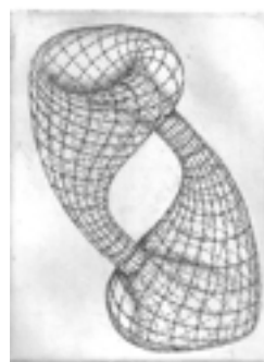
Fig. 15. Double Klein-bottle
