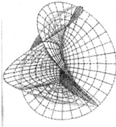
Fig. 13. Henneberg surface
