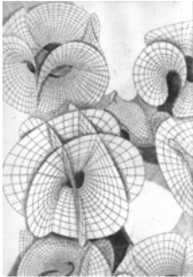
Fig. 11. Floraison
